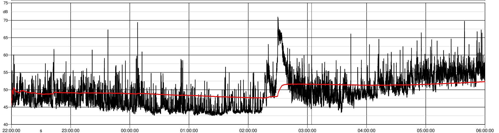
SET_O1 - 5° periodo notturno 1/3 Leq Spectrum + SLM - Min Lineare
