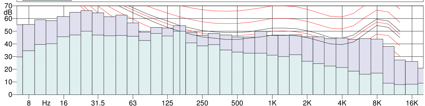
SET_O1 - 7° periodo diurno - 1/3 Leq Spectrum + SLM - Leq - Lineare SET_O1 - 7° periodo diurno - 1/3 Leq Spectrum + SLM - Min - Lineare
