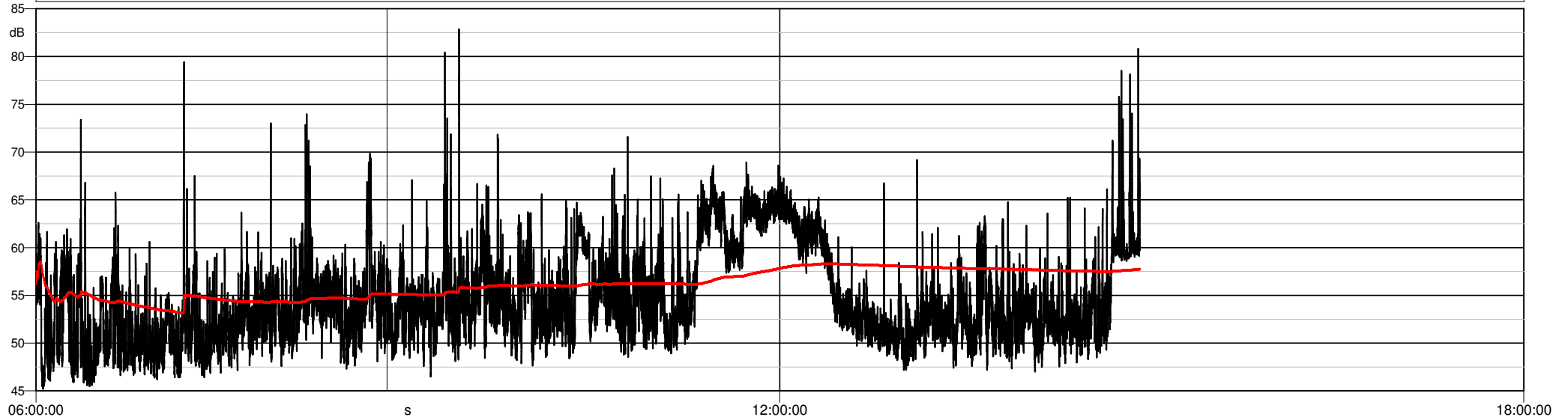
SET_O1 - 7° periodo diurno 1/3 Leq Spectrum + SLM - Min Lineare
