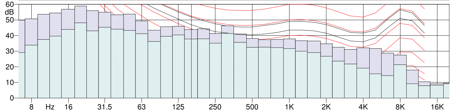
SET_O1 - 1° periodo notturno - 1/3 Leq Spectrum + SLM - Leq - Lineare SET_O1 - 1° periodo notturno - 1/3 Leq Spectrum + SLM - Min - Lineare
