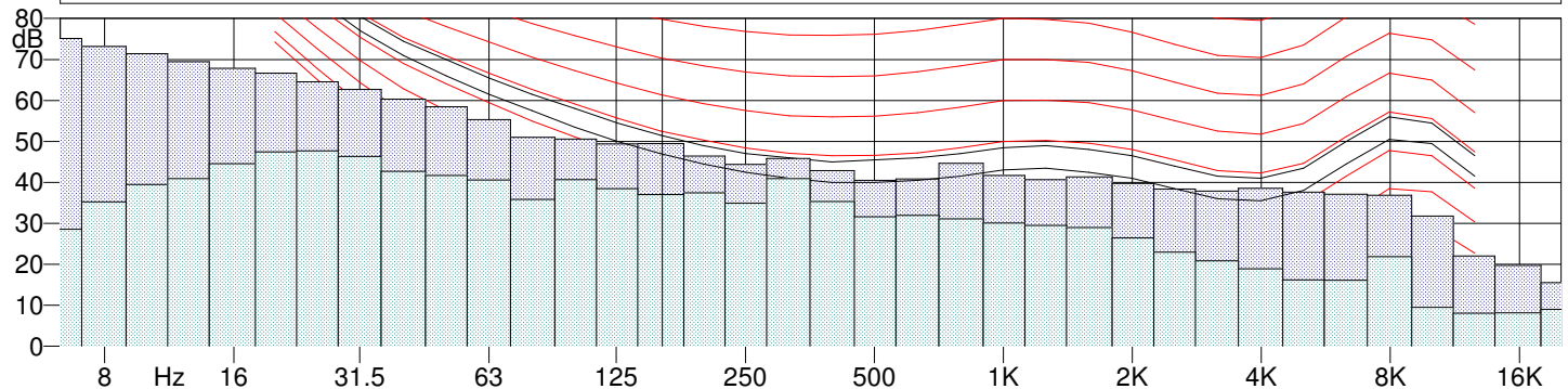
SET_O1 - 5° periodo notturno - 1/3 Leq Spectrum + SLM - Leq - Lineare SET_O1 - 5° periodo notturno - 1/3 Leq Spectrum + SLM - Min - Lineare
