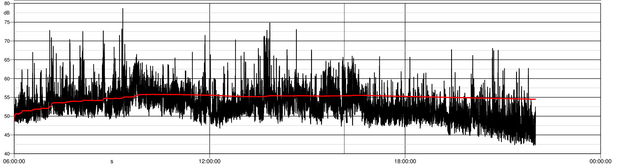
SET_O1 - 6° periodo diurno LAS - Running Leq
