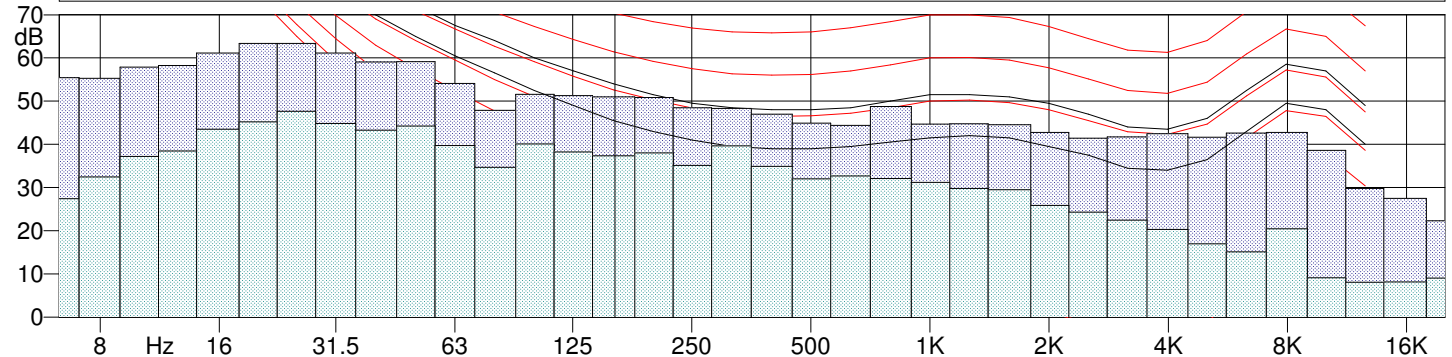
SET_O1 - 2° periodo diurno - 1/3 Leq Spectrum + SLM - Leq - Lineare SET_O1 - 2° periodo diurno - 1/3 Leq Spectrum + SLM - Min - Lineare
